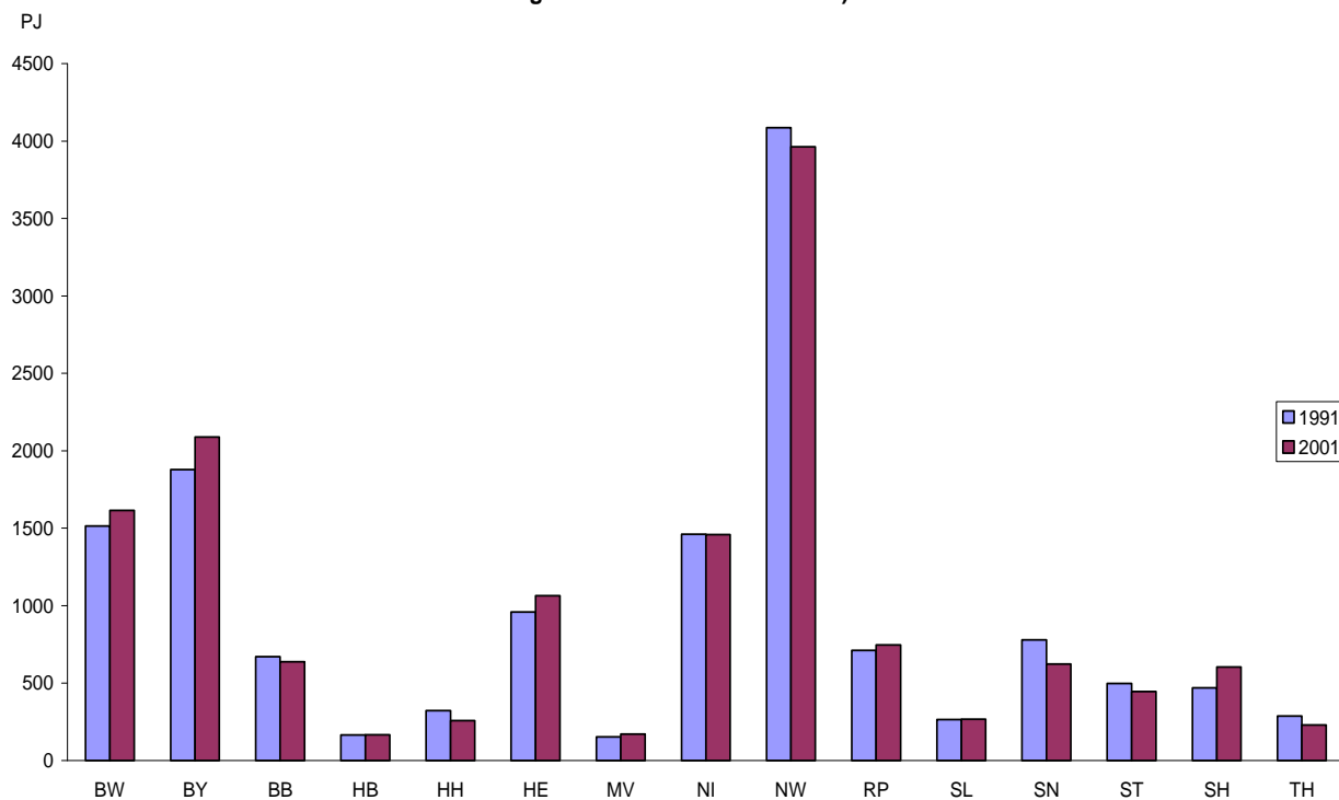
Schaubild 3: Primärenergieverbrauch 1991 und 2001*) nach Bundesländern
