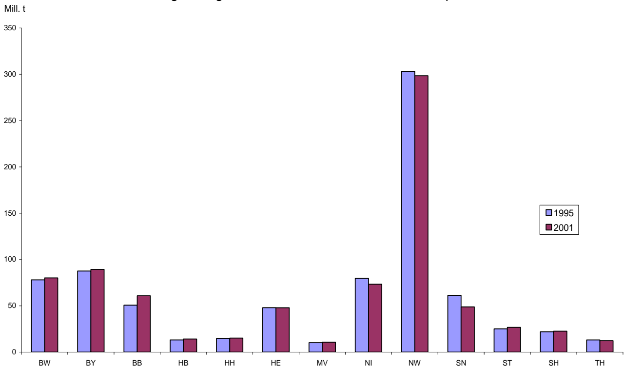
Schaubild 3: Energiebedingte Kohlendioxidemissionen 1995 und 2001*) nach Bundesländern
