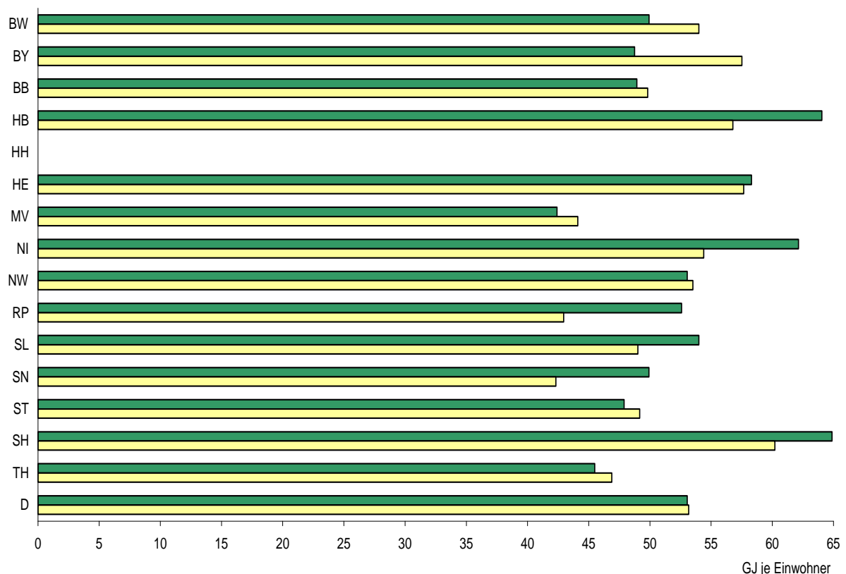
Schaubild 1: Endenergieverbrauch privater Haushalte und Kleinverbraucher je Einwohner 1991 und 2001* nach Bundesländern
