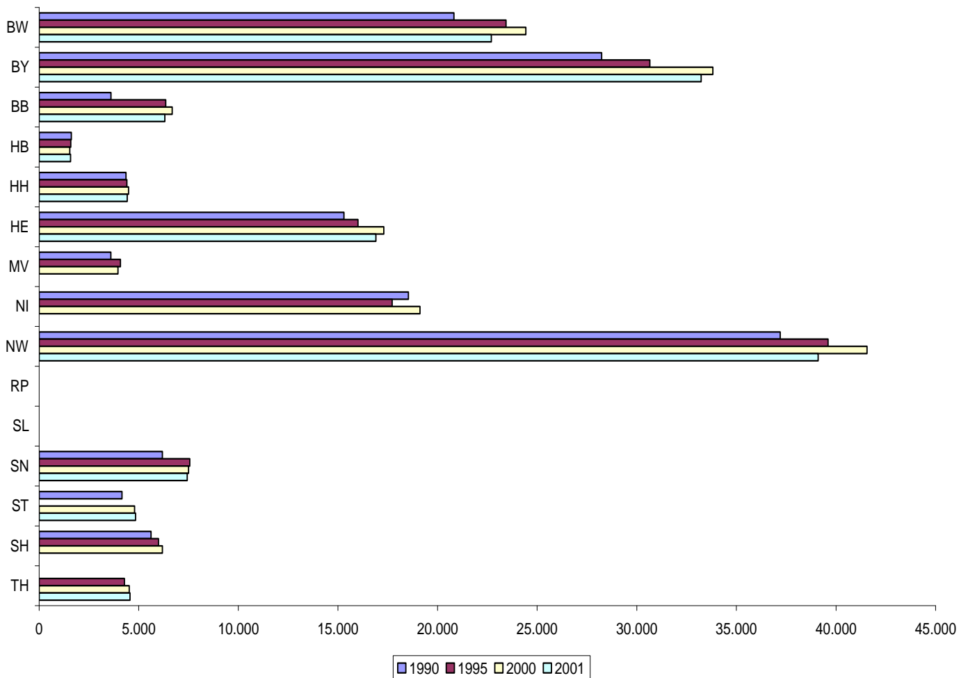
Schaubild 1: Jährliche CO 2 -Menge des Verkehrs in 1000 to/a
