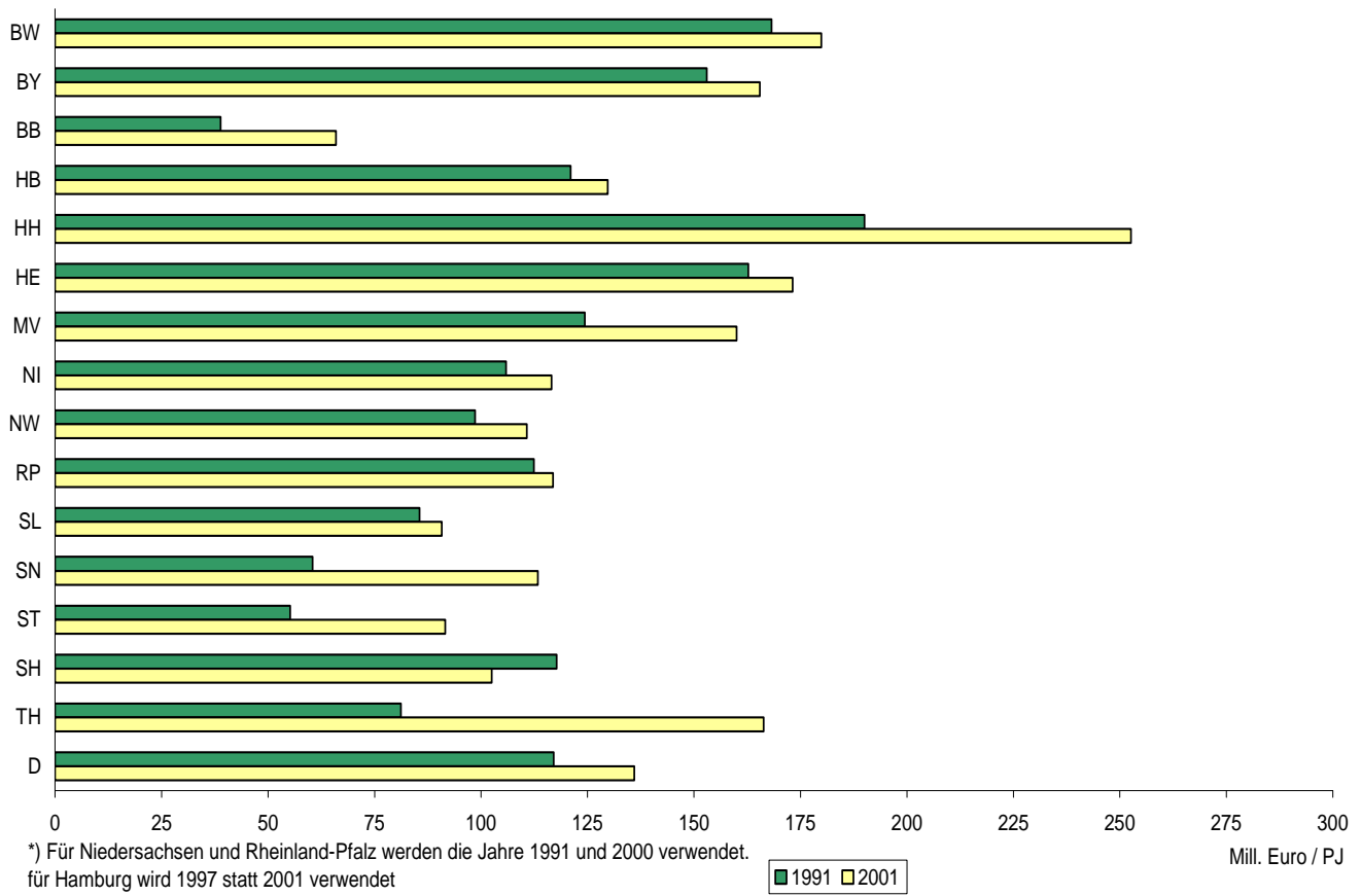
Schaubild 1: Energieproduktivität 1991 und 2001*) nach Bundesländern
