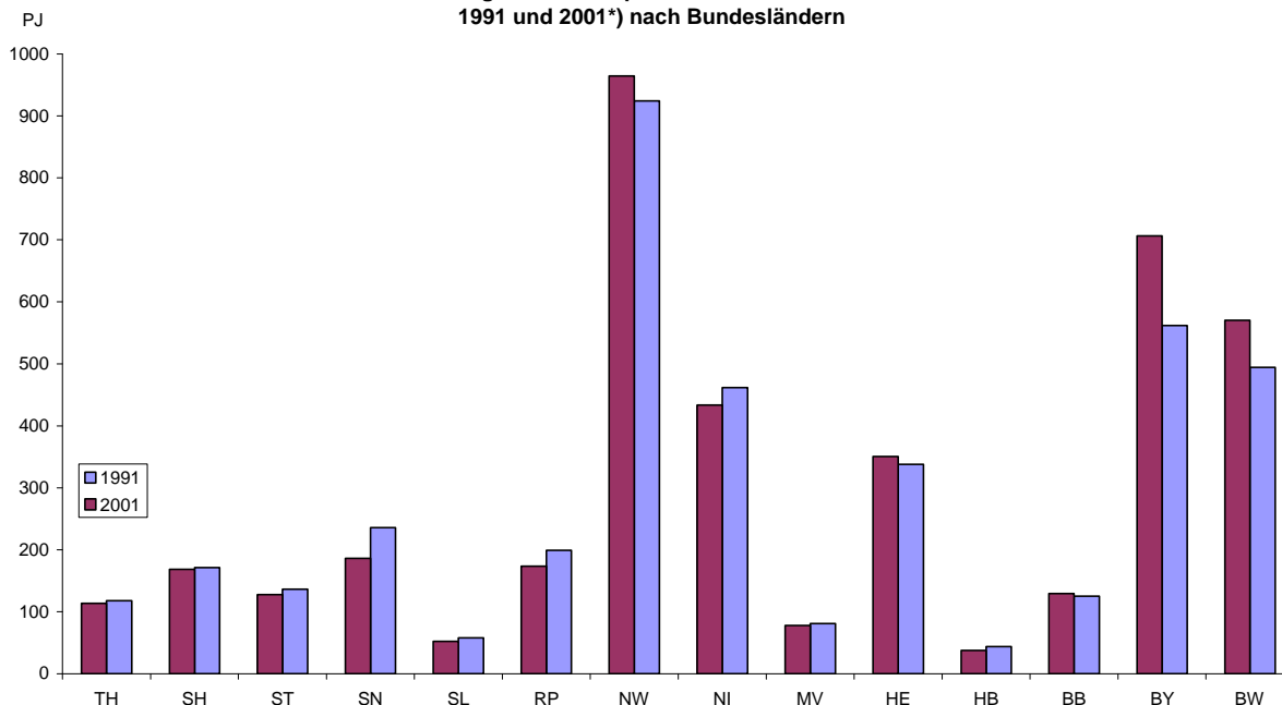
Schaubild 3: Endenergieverbrauch privater Haushalte und Kleinverbraucher 1991 und 2001*) nach Bundesländern
