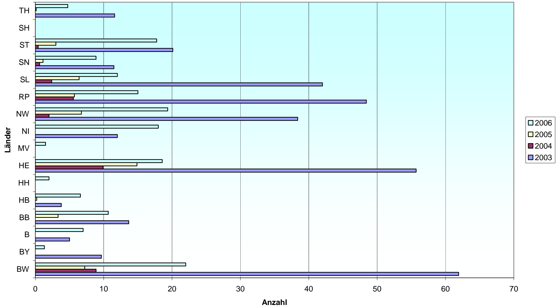
Ozon: Zahl der Stundenwerte > 180 µg/m 3 im Mittel über alle Stationen des Typs "städtischer Hintergrund"
